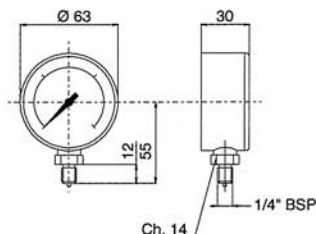
Radiale / Radial MAR-63
